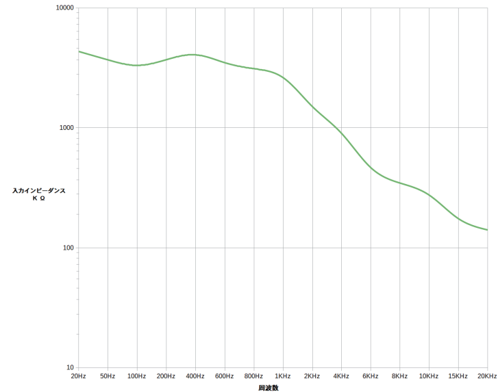
CURVED II 入力インピーダンス ※計算値
